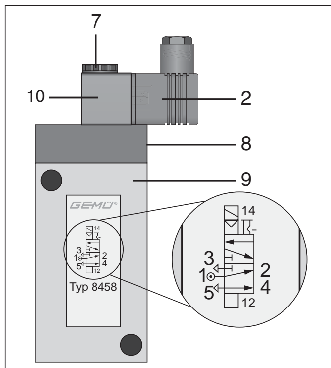
Geräteaufbau
