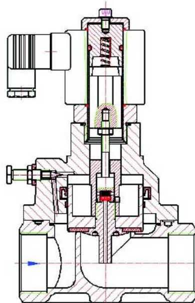
Baureihe 49
